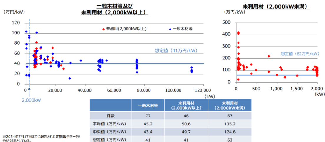
【参考 63】一般木材等・未利用材バイオマス発電の資本費
