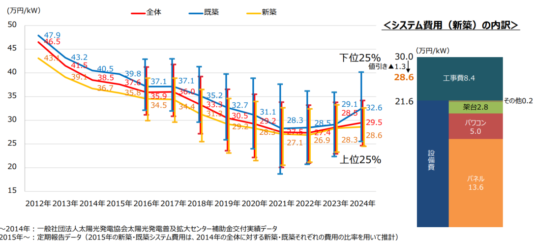
【参考 18】住宅用太陽光発電のシステム費用の推移とその内訳
