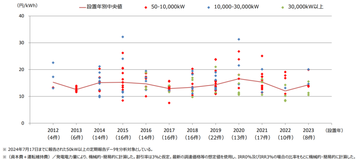
【参考 34】陸上風力発電の設置年別の kWh 当たりの発電コスト
