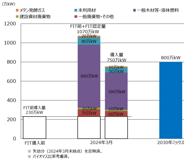
【参考 58】 バイオマス発電の年度別・規模別の FIT・FIP 認定量
