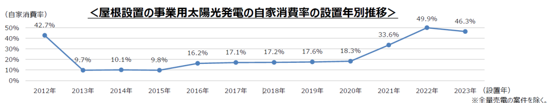
【参考 14】 事業用太陽光発電（屋根設置）の自家消費率の設置年別推移
