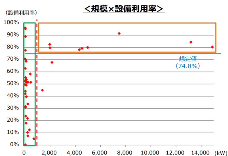
【参考 47】地熱発電の出力と設備利用率の関係
