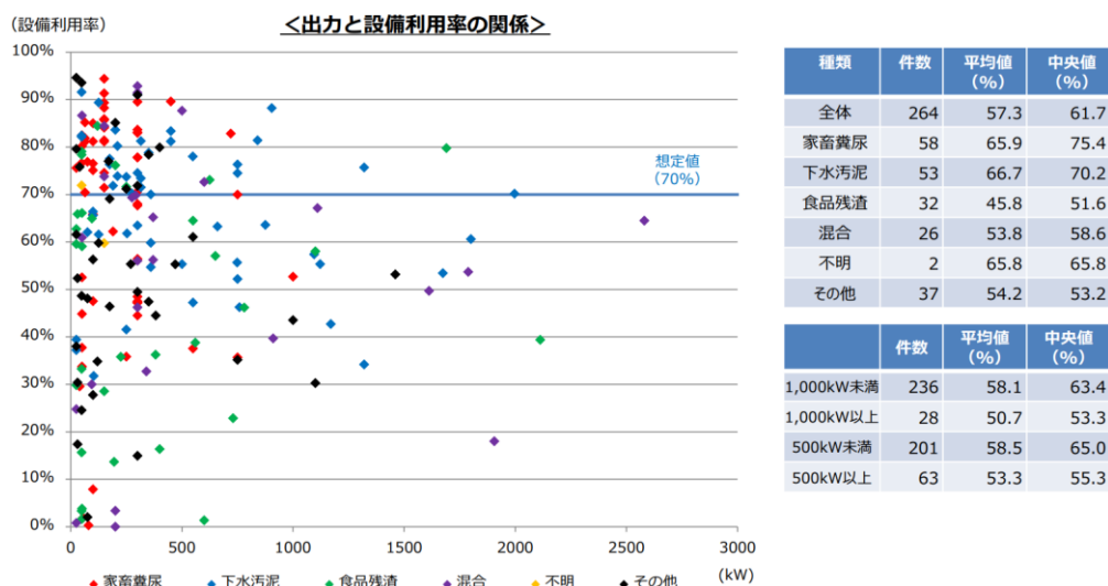
【参考 73】メタン発酵バイオガス発電の設備利用率
